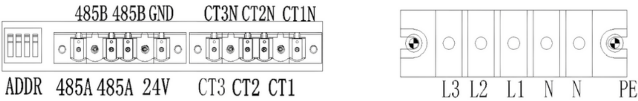
Rysunek 2. Widok złączy oraz wejść kompensatora.
